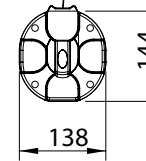
Installazione frontale Head-on installation
