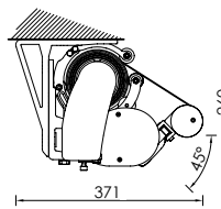
Installazione a soffitto 45° Ceiling installation 45°
