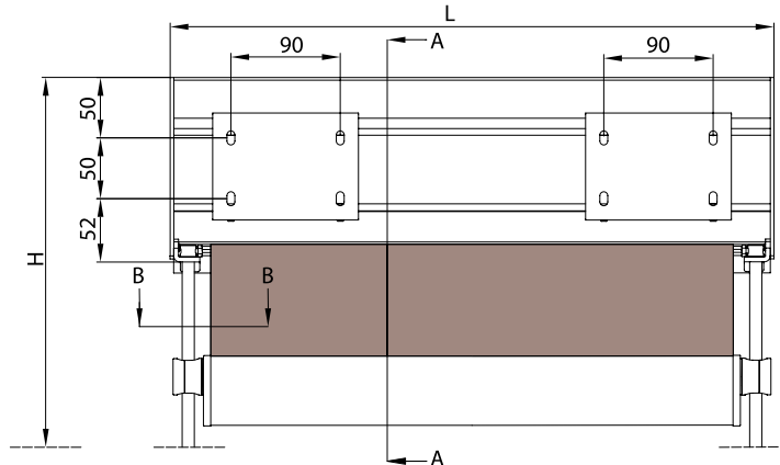
supporto a parete - wall bracket
