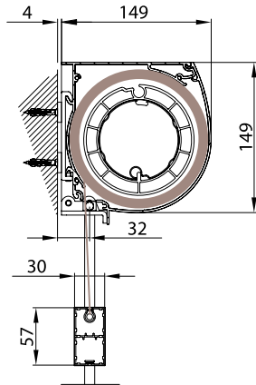
TONDO - ROUND A-A
