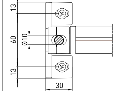
pedino a pavimento - floor bracket B-B
