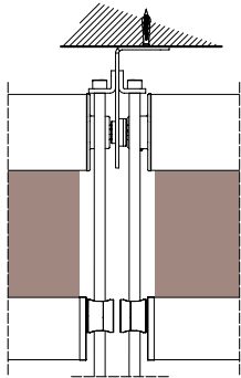
modulo doppio double module A-A
