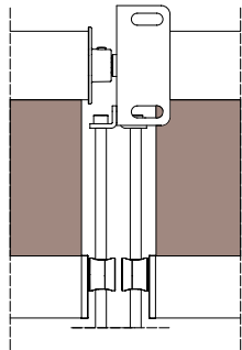
modulo doppio double module A-A
