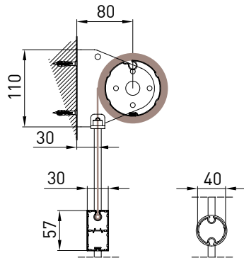
GA Posteriore - GA back A-A
